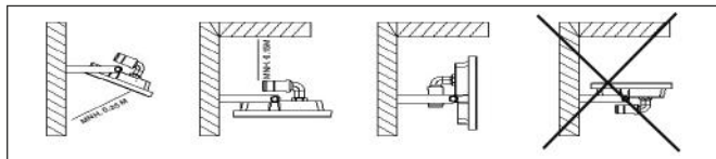
Fig.2: Montageort
